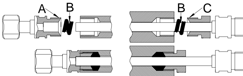
Bild 4: Aufbau Absaugrohre mit auswechselbarem Innenrohr.
