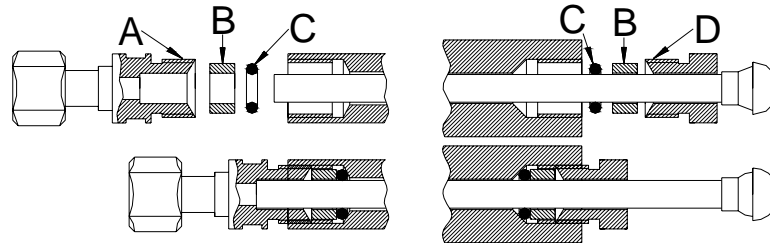
Bild 5: Aufbau Absaugrohre mit auswechselbaren Innenrohren.
